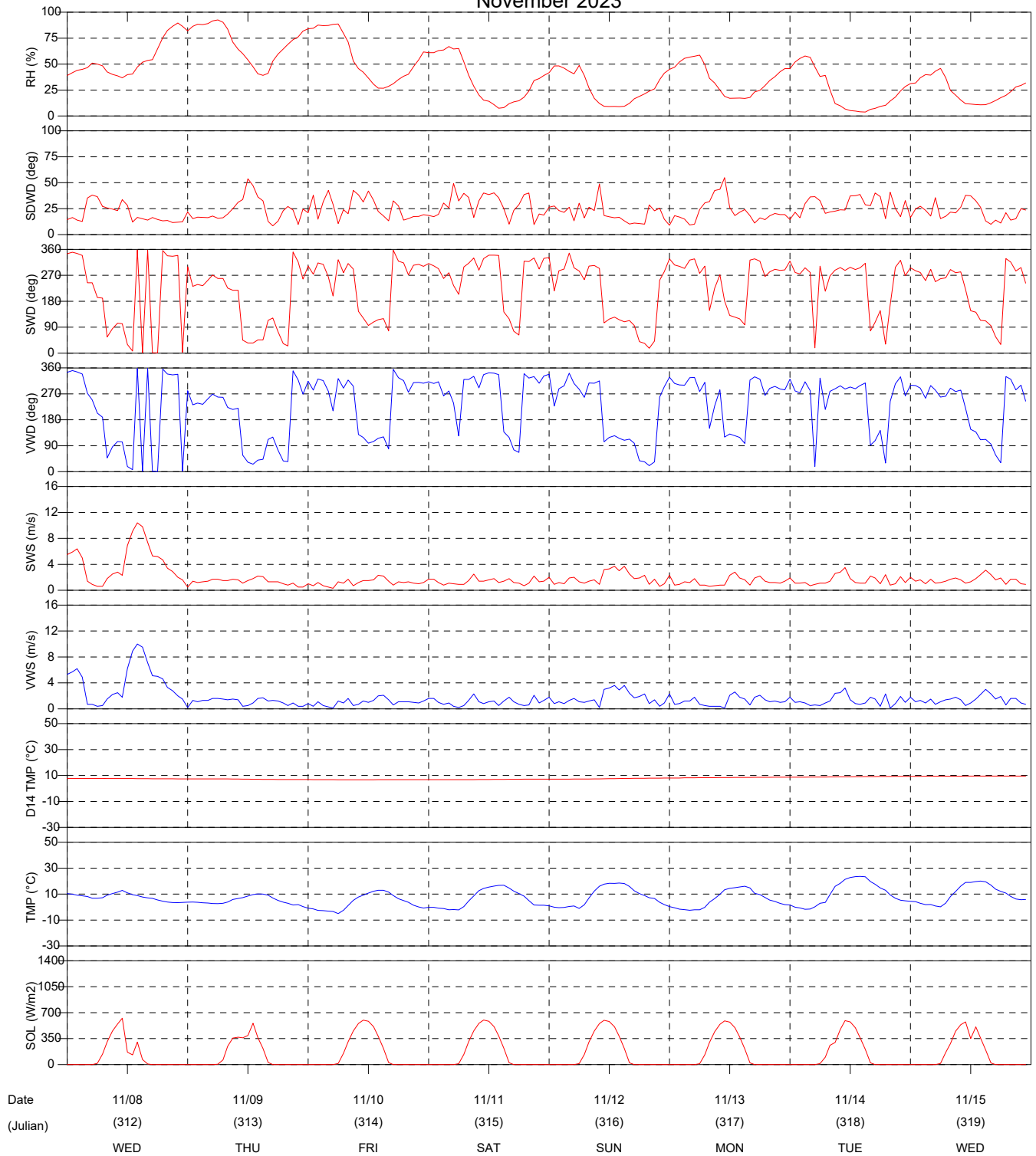
Figure 4-13 Colorado Air Toxics - C1 (Pueblo) - Hourly Met Data November 2023
