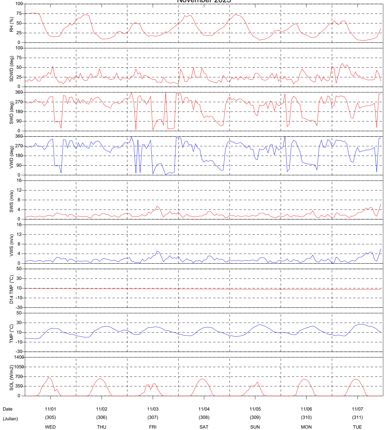
Figure 4-12 Colorado Air Toxics - C1 (Pueblo) - Hourly Met Data November 2023
